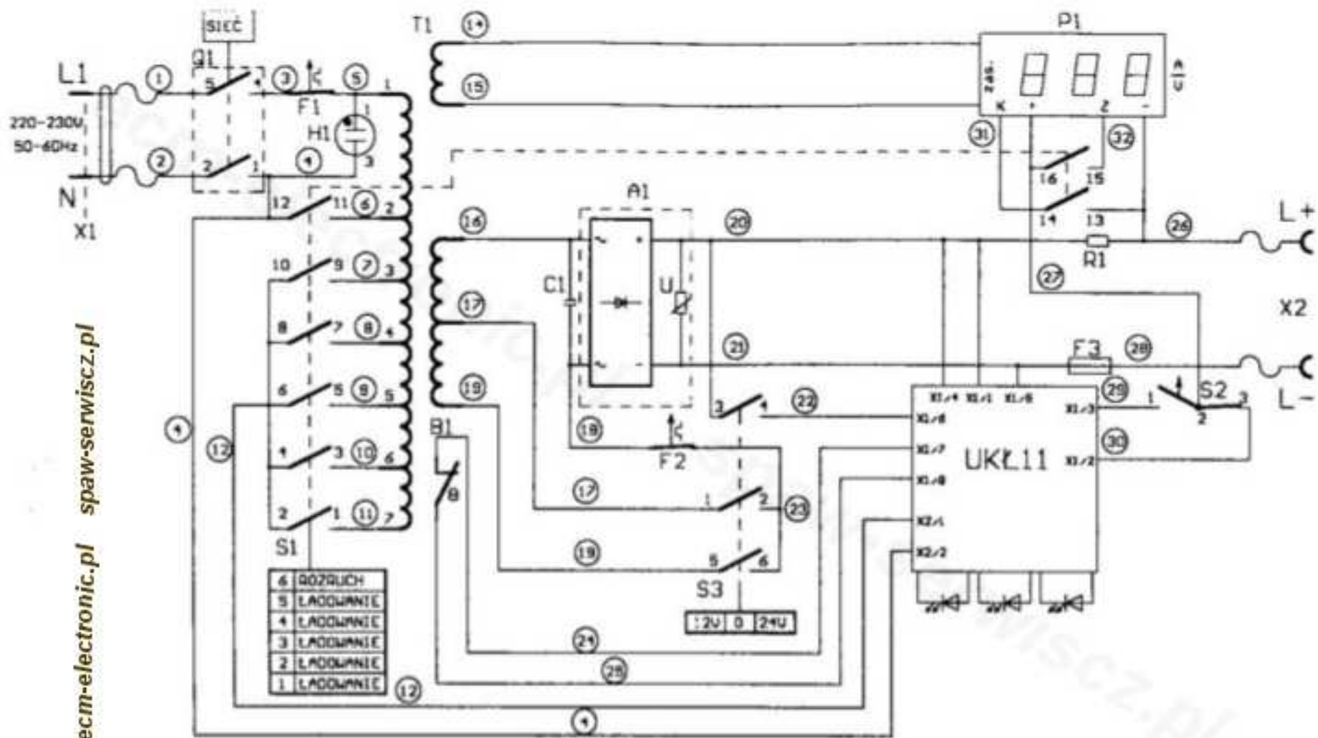
Schemat ideowy zespołu prostownikowego HERKULES 300
