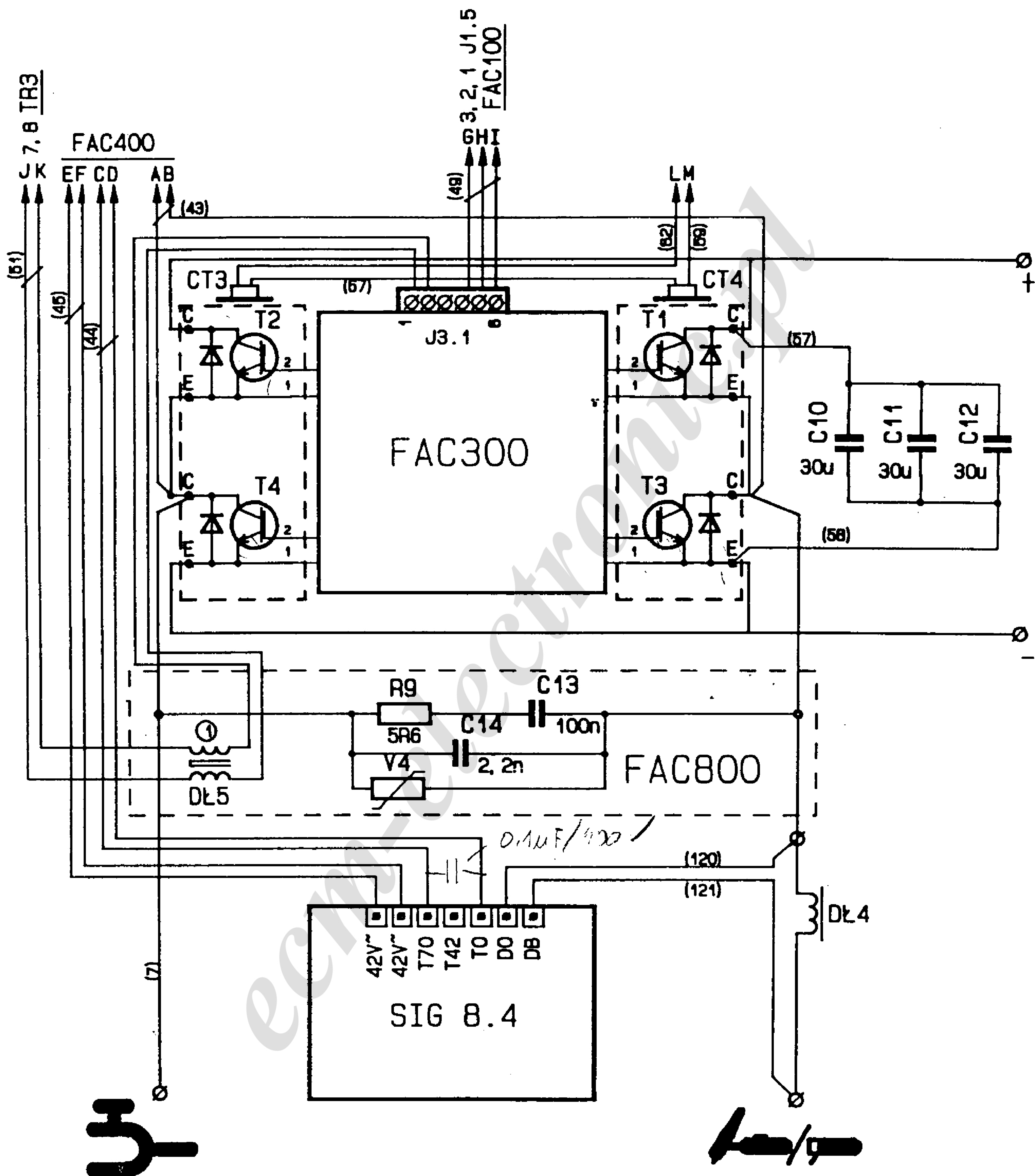
Urządzenie FALTIG-315 AC/DC schemat ideowy 02
