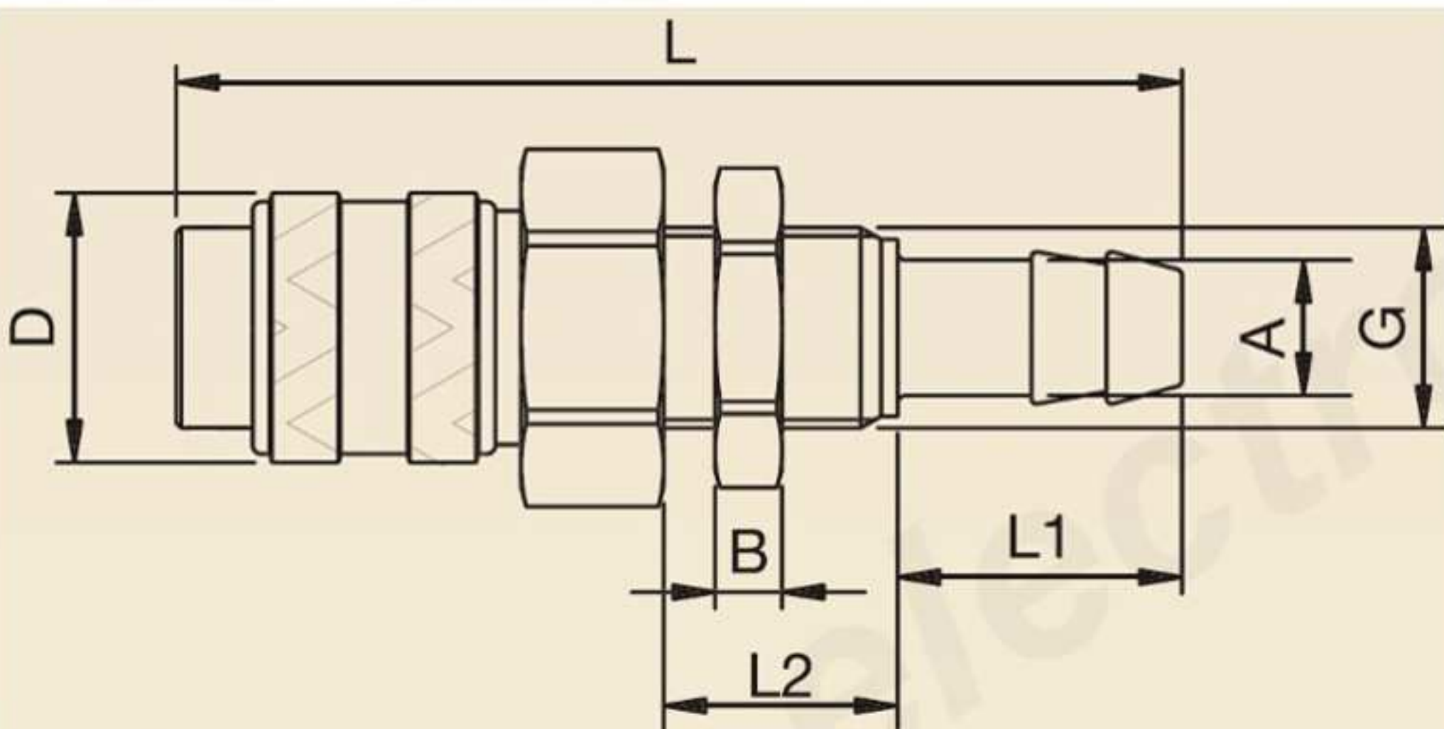
Szybkozłączki - gniazda - montaż panelowy, tuleja do węża - Typ 21KA zamienniki
